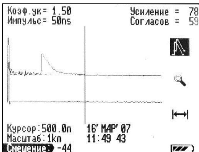
Рисунок 6-12 Режим сравнения с памятью
