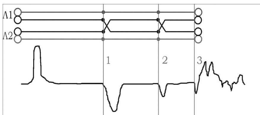
Рисунок 6-8 «Разбитость пар»
