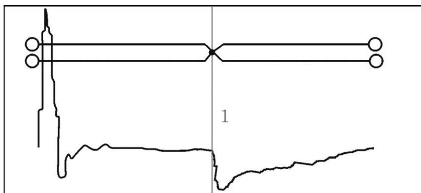
Рисунок 6-5 Короткое замыкание
