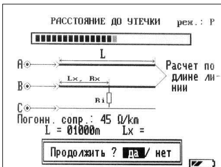
Рисунок 4-6 Вид дисплея в режиме «Повреждение», пункт «Утечка»
