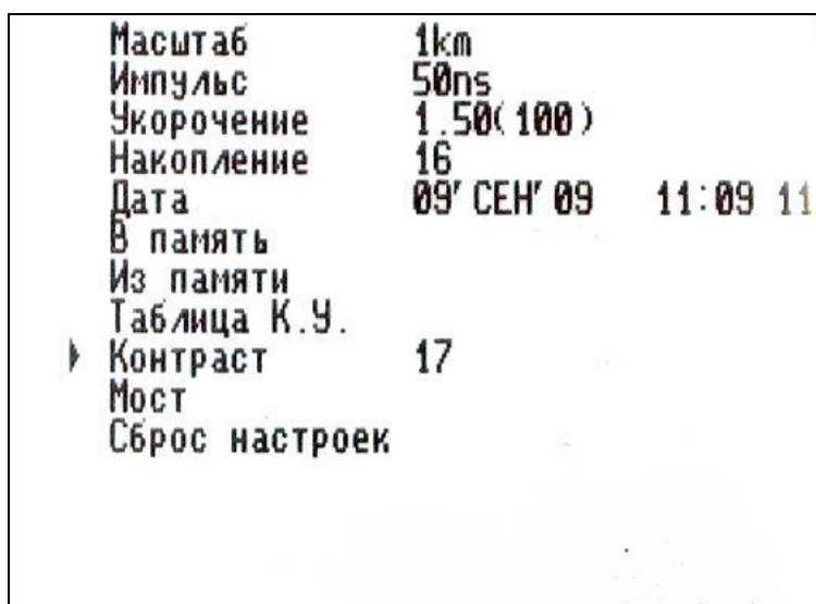
Рисунок 4-4 Вид дисплея в режиме МЕНЮ рефлектметра
