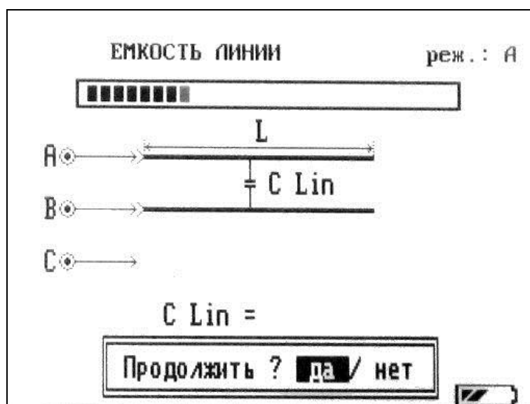
Рисунок 6-16 Измерение ёмкости линии
