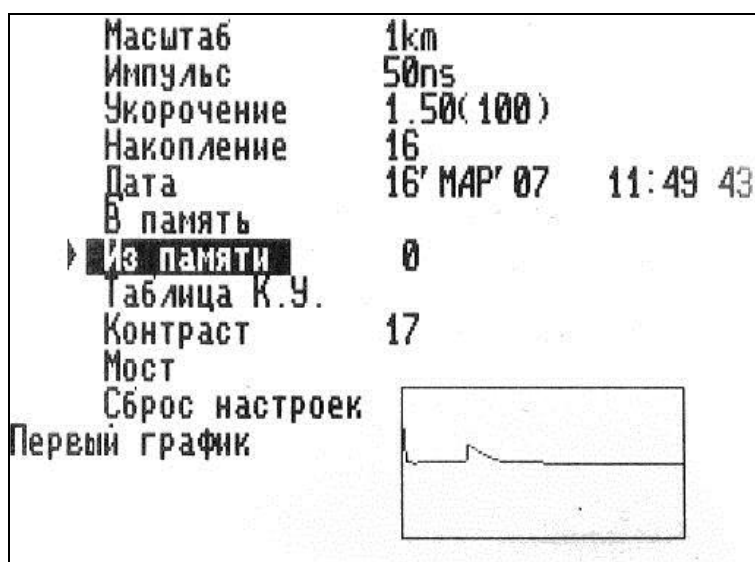
Рисунок 6-11 Вывод рефлектограммы из памяти
