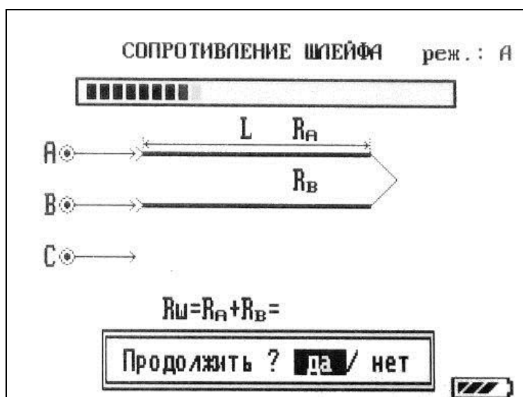
Рисунок 6-14 Измерение сопротивления шлейфа
