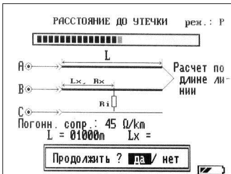
Рисунок 6-17 Метод Муррея
