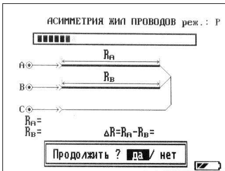
Рисунок 6-15 Измерение асимметрии жил проводов
