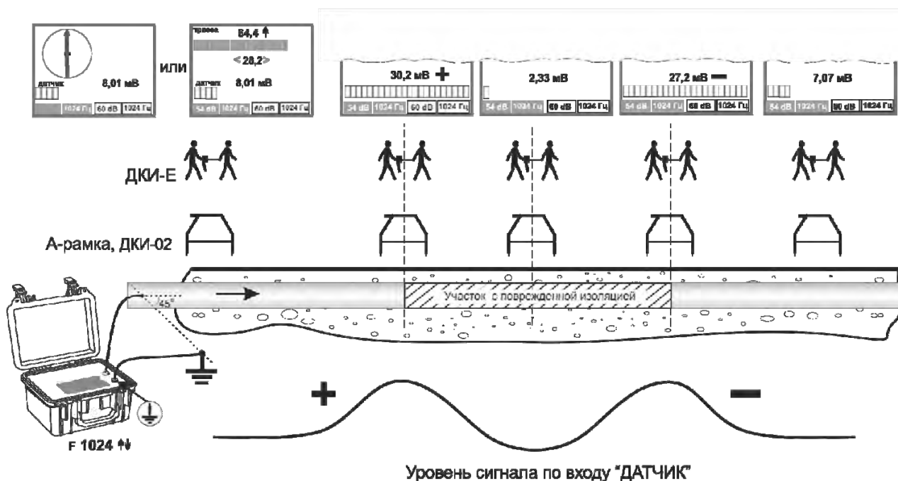
Рисунок 5.2.1 – Схема подключения и уровень сигнала при поиске повреждения изоляции по падению сигнала со сменой знака
