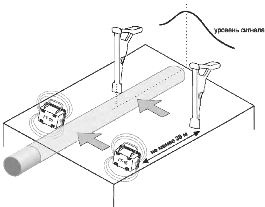
Рисунок 4.4.2 б – Обследование участков местности с помощью ГТ-15
