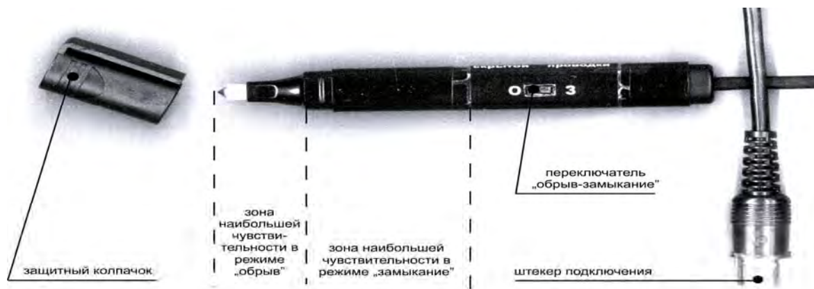
Рисунок 5.3.4.1 – Мини-датчик МД-01
