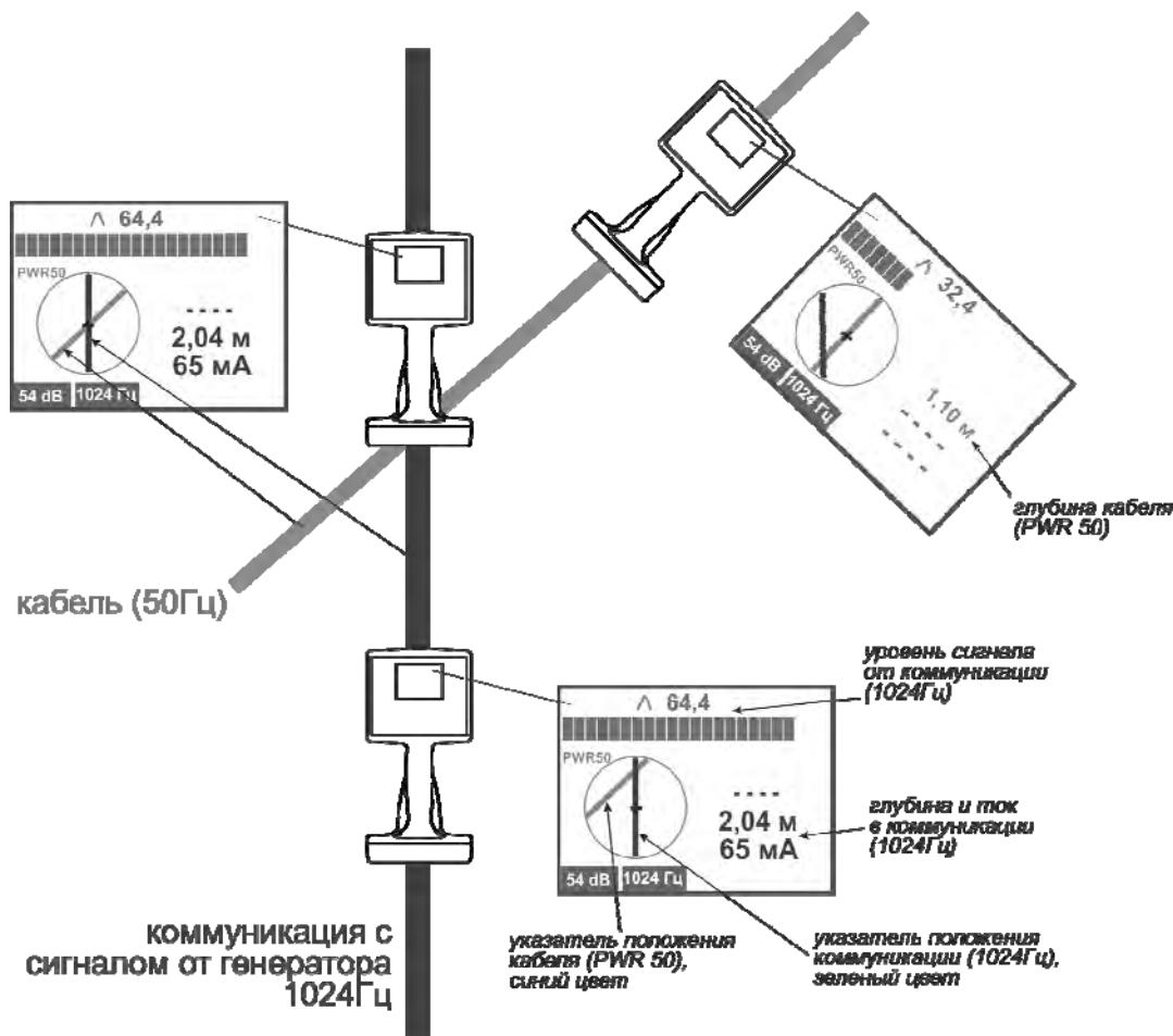
Рисунок 4.2.3б – Поиск с включенной функцией «Вторая линия»
