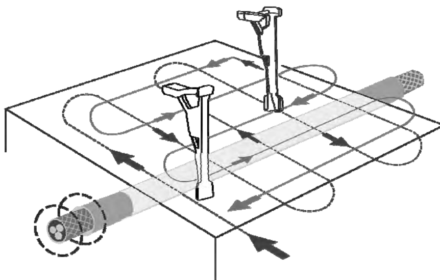
Рисунок 4.4.1 – Обследование участков местности без генератора
