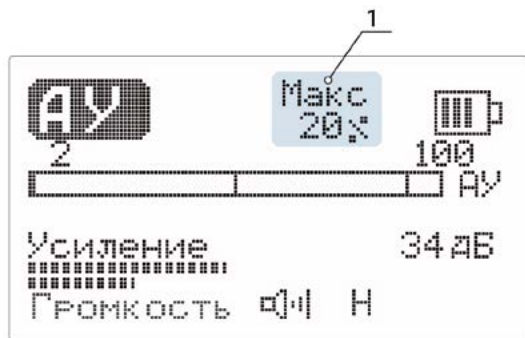
Рисунок 8 – Основной экран канала «АУ»
