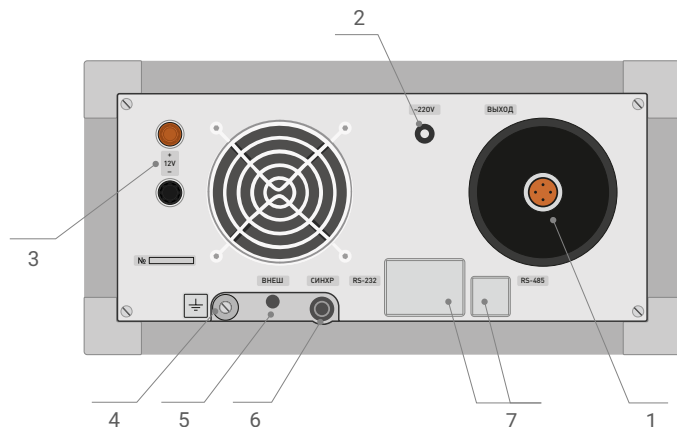
Рисунок 2 - Задняя панель генератора
