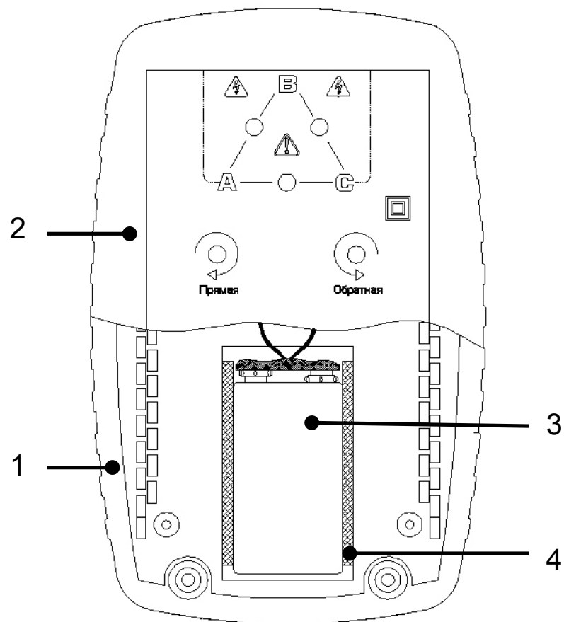
Рисунок 4.2 – Расположение батареи в указателе
