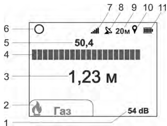
Рисунок 3.2а – Вид индикатора в режиме поиска одного типа маркера, где:
